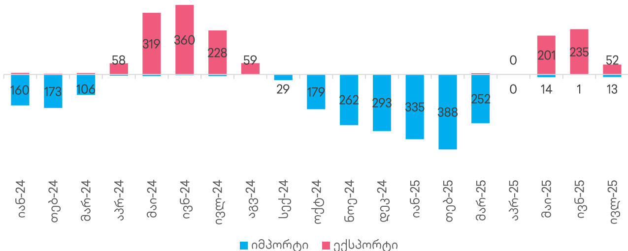
გრაფიკი 4. ელექტროენერჯის იმპორტი და ექსპორტი, გვტ. საათი
